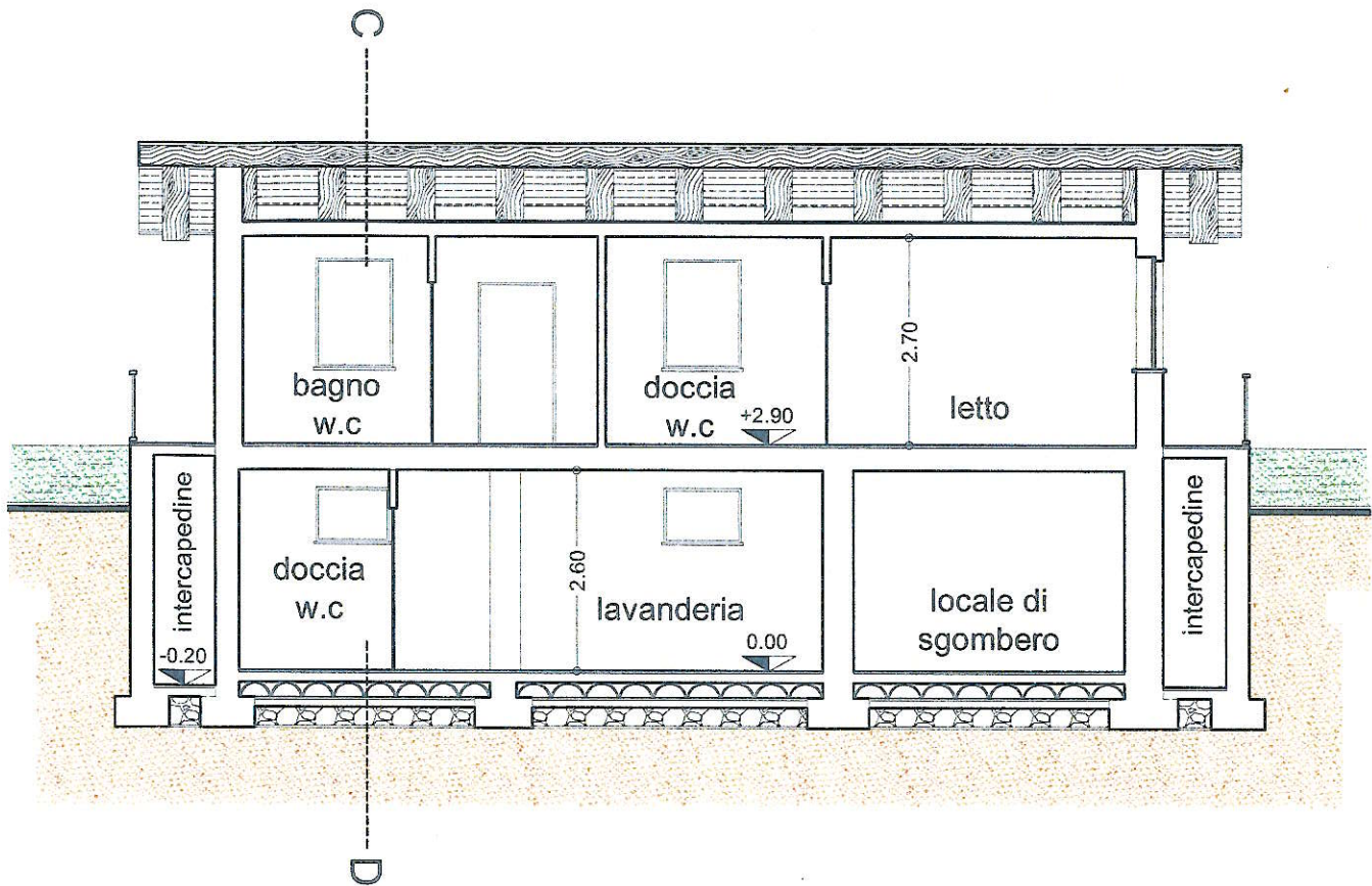
SEZIONE A - B scala 1:100
