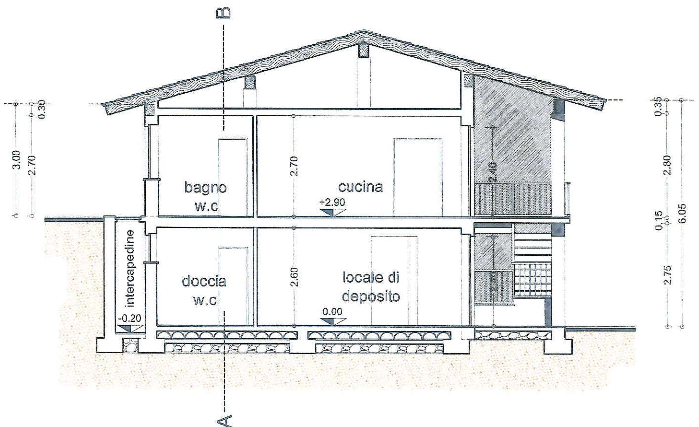
SEZIONE C - D scala 1:100
